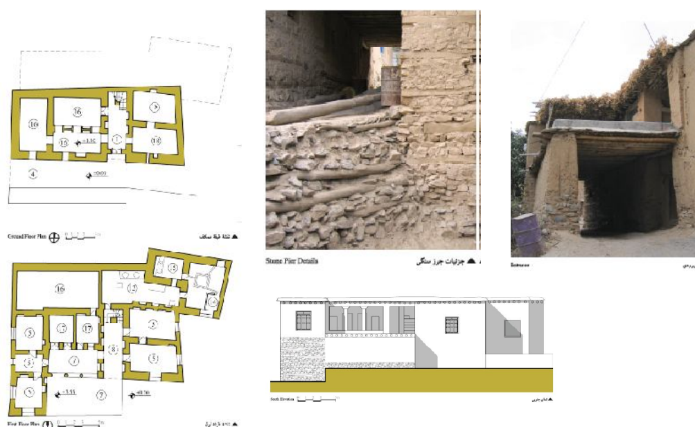
1. ورودی، 4. دالان، 5. اتاق، 7. ایوان، 8. راهرو، 13. آشپزخانه، 14. دستشویی، 15. حمام، 16. انبار، 17. دستشویی، 18. طویله
