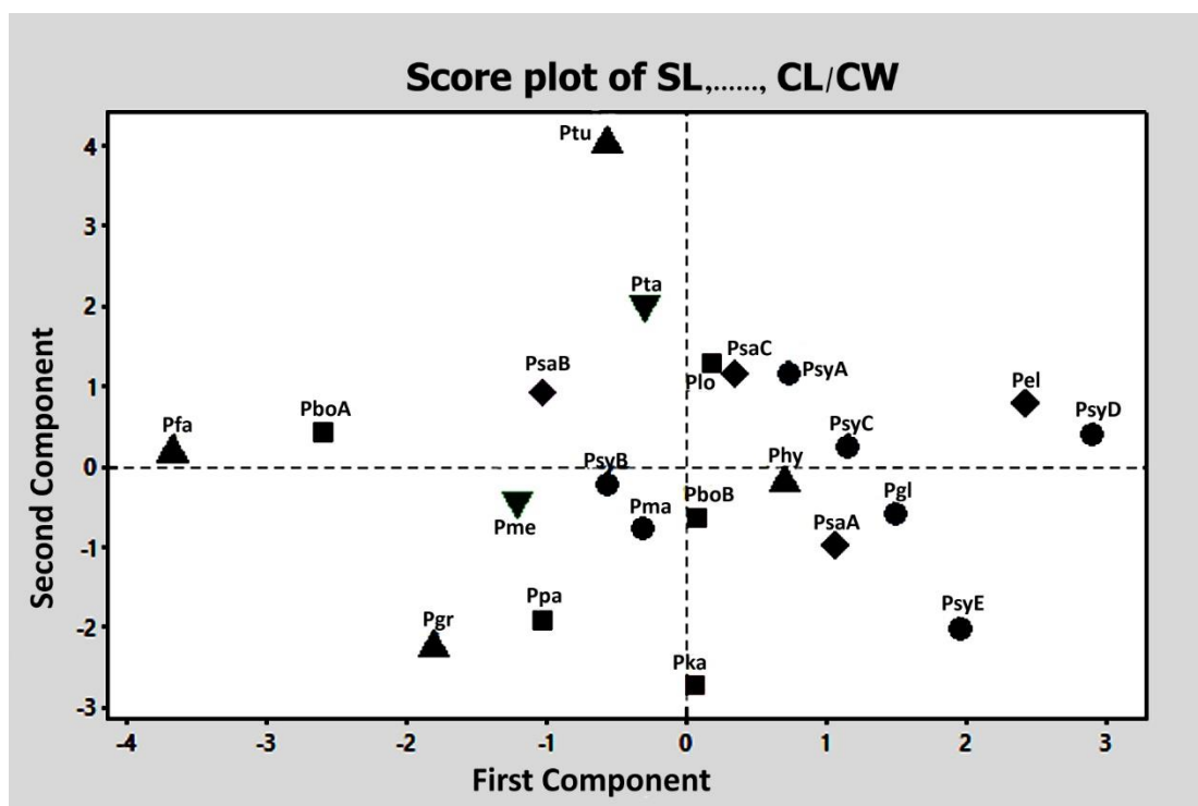
شکل ۳- رسته‌بندی PCA آرایه‌های مختلف گلابی بر اساس مطالعه ریزریخت‌شناسی بذر (■: بخشه Pashia ; ▲: بخشه Pyrus ; ●: بخشه Xeropyrenia ; ◆: بخشه Argyromalon ; ▼: آرایه‌های دورگه).
