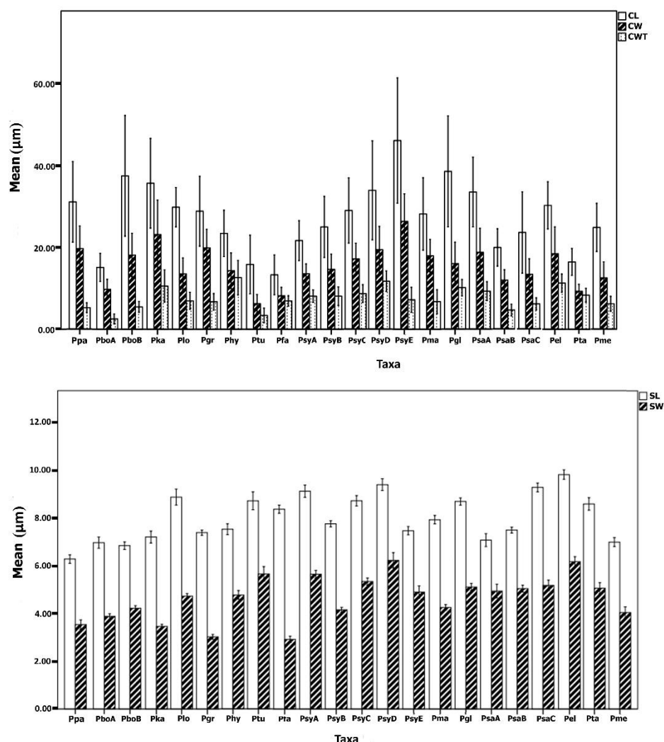
شکل ۲- میانگین و انحراف معیار پنج صفت کمی مورد مطالعه در ریزریخت‌شناسی بذر آرایه‌های گلایی شامل طول بذر (SL)، عرض بذر (SW)، طول سلول سطحی بذر (CL)، عرض سلول سطحی بذر (CW)، ضخامت دیواره سلول سطحی بذر (CWT).
