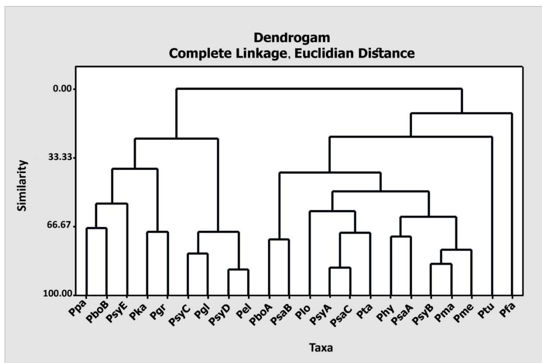
شکل ۴- دندروگرام حاصل از آنالیز خوشه‌ای آرایه‌های مورد مطالعه گلابی بر اساس صفات کمی بذر با استفاده از روش همبستگی کامل و فاصله اقلیدسی.
