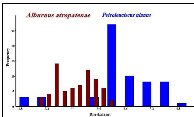
شکل ۳- تحلیل تابع تشخیصی (DFA) دو گونه A. atropatenae و P. ulanus بر اساس صفات اندازه‌شی.
