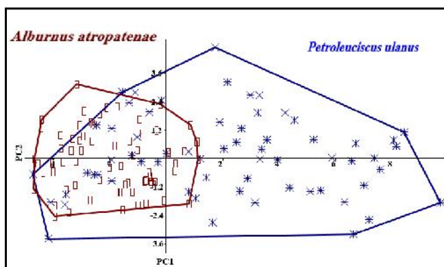
شکل ۲- نمودار تجزیه به مولفه‌های اصلی (PCA) دو گونه A. atropatenae و P. ulanus بر اساس صفات اندازه‌شی.
