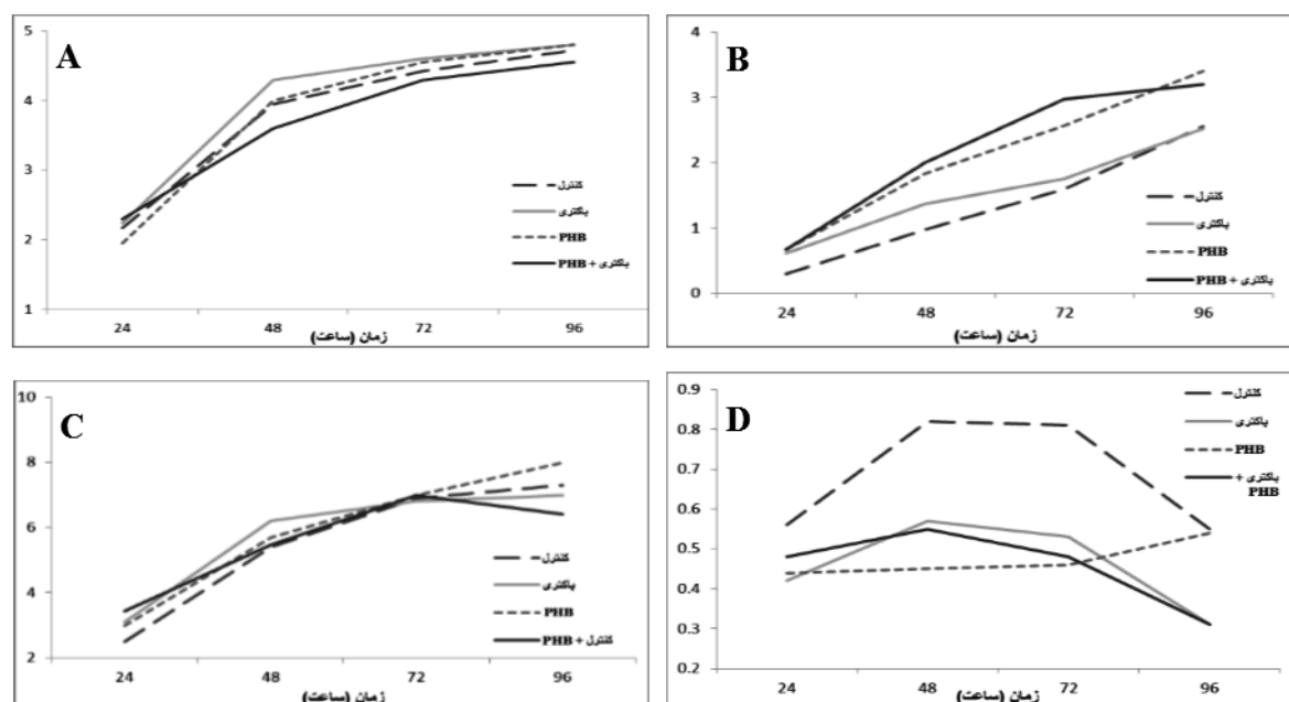
شکل ۲- A. استفاده از منابع کربنی پلیمری. B. اسید آمینه ای. C. کربوهیدرات. D. کربوکسیلیک اسید به وسیله باکتری‌های غیرهوازی قابل کشت در انتهای روده بچه ماهیان تاسماهی سبیری.
