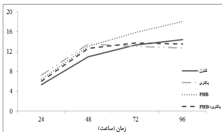
شکل ۱- منحنی میانگین فعالیت رنگ (AWCD) یا فعالیت متابولیکی باکتری‌های بی‌هوازی در روده بچه ماهیان تاسماهی سبیری تغذیه شده با تیمارهای غذایی در طول ۹۶ ساعت دوره انکوباسیون و ۲۵ درجه سانتیگراد.
