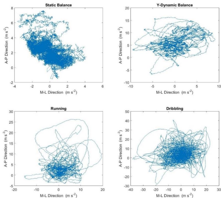
شکل ۲. تغییرات شتاب در راستاهای میانی جانبی و قدامی خلفی در آزمون‌های تعادل ایستا، پویا، دویدن و در بیل‌زدن
