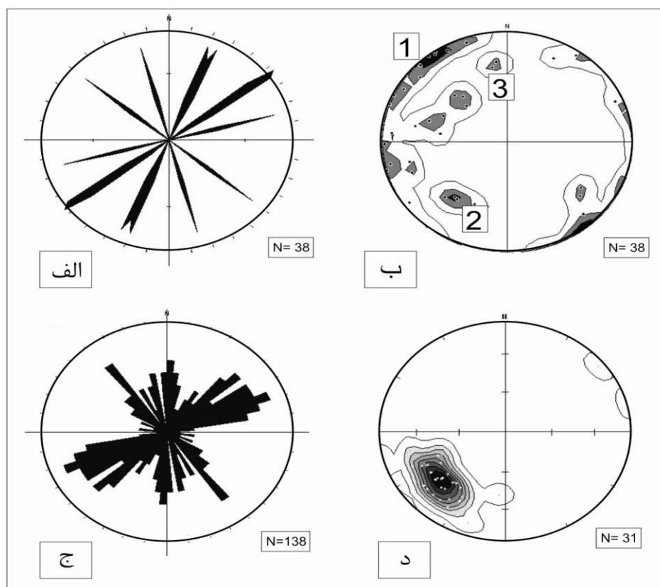
شکل ۳. الف) پراکندگی آماری گسل‌های منطقه بر روی نمودار گلسرخی، ب) پراکندگی آماری گسل‌های منطقه روی نمودار استریونوت هم مساحت، شماره ۱، ۲ و ۳ به ترتیب نقاط تجمعی بیش‌ترین پراکندگی و سامانه‌های مختلف گسلی مطالعه شده را نشان می‌دهد، ج) نمودار گلسرخی حداکثر درزه و شکستگی‌های موجود در سنگ‌های منطقه، د) نمودار استریونوتی هم مساحت شیستوزیته‌های برداشت شده سنگ‌های منطقه
