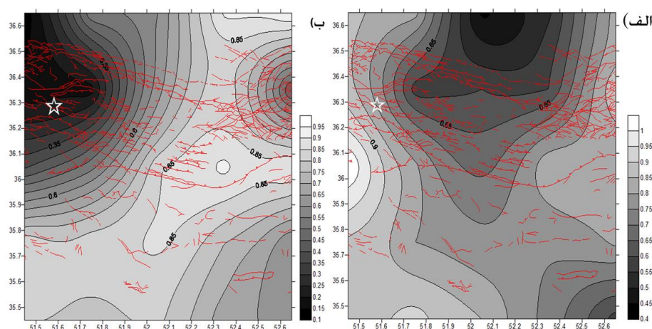
شکل ۸. نقشه‌های تغییرات مکانی D_e : الف) قبل از زمین‌لرزه، ب) بعد از زمین‌لرزه. خطوط قرمز گسل‌ها (برگرفته از سازمان زمین‌شناسی و اکتشاف معدنی کشور)، ستاره روکانون زمین‌لرزه
