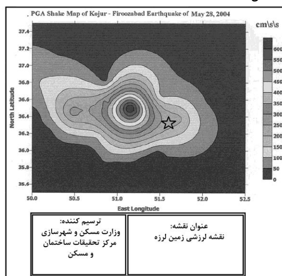
شکل ۱۰. نقشه لرزشی زمین‌لرزه بلده-کجور (برگرفته از گزارش شماره ۲ مرکز تحقیقات ساختمان و مسکن) با توجه به این نکته که b-value مربوط به لرزه‌خیزی پس‌زمینه که پس از حذف خوشه‌های لرزه‌ای به‌دست می‌آید، می‌تواند محل تنشگاه‌ها را نشان دهد، این خوشه‌ها (پیش‌لرزه و پس‌لرزه) از بین داده‌ها حذف شد. سپس نقشه
