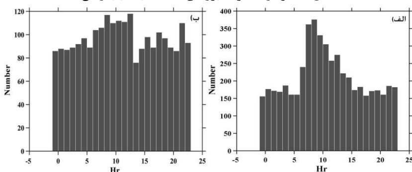
شکل ۳. هیستوگرام تعداد زمین‌لرزه‌ها در ساعات شبانه روز: الف) برای زمین‌لرزه‌های با M \geq 1.7 و ب) M \geq 2.1
