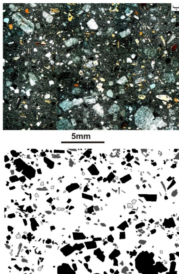
شکل ۴. تصویر مقطع KHD7 به همراه تصویر بلورهای پردازش شده پلاژیوکلاز (مشکی)، آمفیبول (خاکستری تیره) و کوارتز (خاکستری روشن)
