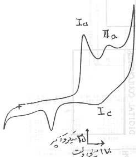
شکل ۳: ولتاموگرام چرخه‌ای محلول 24 gr/l پوسته خارجی برنج در الکترولیت 5M H_2SO_4 و در حضور 0.01M Ce(IV) ، Pt الکترود آند. سرعت جاروب 30mv/sec. محدوده پتانسیل ۱.۰۵ تا ۱.۵۵ میلی‌ولت.
