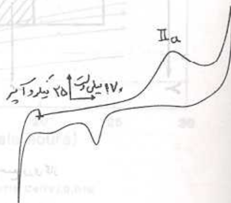
شکل ۲: ولتاموگرام چرخه‌ای محلول 5M H_2SO_4 و در سطح الکترود Pt. محدوده پتانسیل ۱.۰۵ تا ۱.۵۵ میلی‌ولت. سرعت جاروب 30mv/sec.
