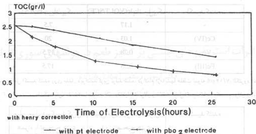
شکل ۴: نمودار تغییرات TOC (gr/l) بر حسب زمان الکترولیز در سطح الکترودهای جامد مختلف.
