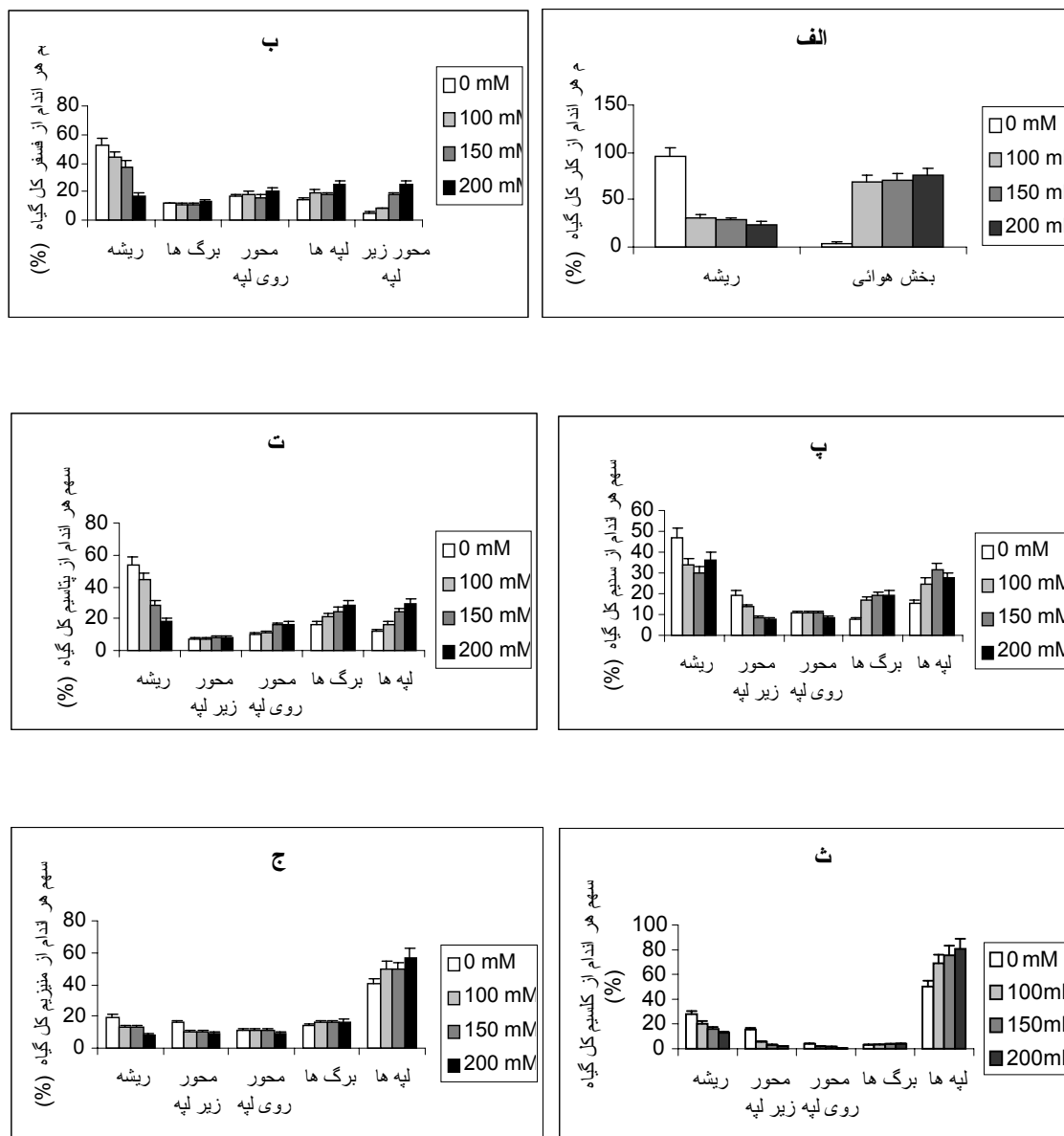
شکل ۲- معرفی سهم هر اندام از مقدار کلر (الف)، فسفر (ب)، سدیم، (پ)، پتاسیم (ت)، کلسیم، (ث) و منیزیم (ج) موجود در کل دانه‌رست‌هائی که جوانه زنی و رشد را به مدت ۱۴ روز در آب مقطر سپری نموده و روز پانزدهم را در محلول‌های هوگلند یک سوم تراکمی، با غلظت‌های مختلف کلرور سدیم (۰، ۱۰۰، ۱۵۰ و ۲۰۰ میلی‌مولار) گذرانده‌اند.
