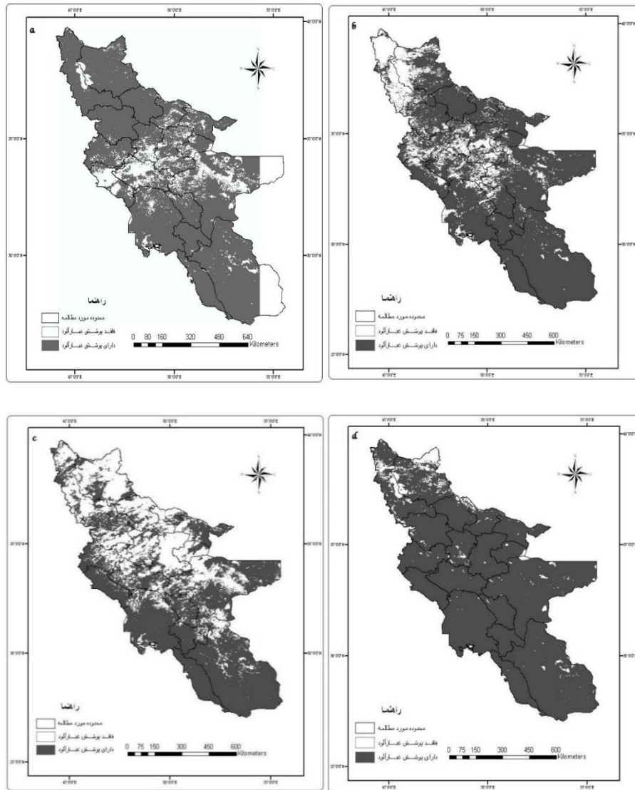
شکل (۵). نقشه‌های نهایی (reclass) حاصل از بکارگیری شاخص NDDI بر روی تصاویر روزهای (a): اول، (b): دوم، (c): سوم و (d): چهارم جولای ۲۰۰۸
