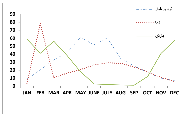
شکل (۳). توزیع ماهانه دما، بارش و روزهای همراه با گرد و غبار در غرب کشور
