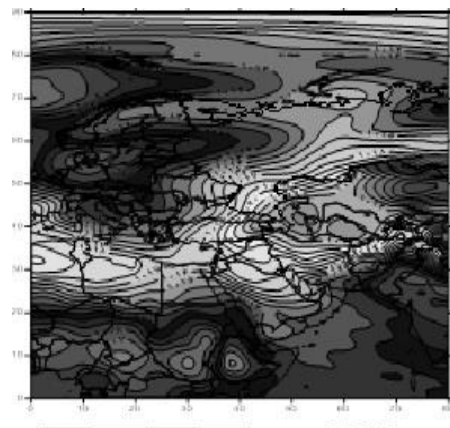
شکل (۶) نقشه سطح دریا slp الگوی پنجم
