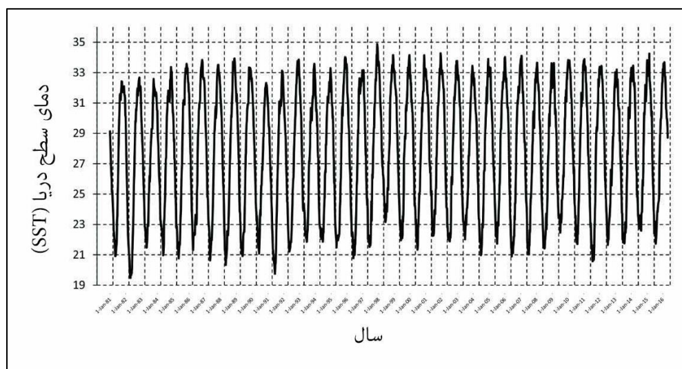
شکل (۴): تغییرات دمای سطح دریا SST شمال خلیج فارس (۱۹۸۰-۲۰۱۴). (کبری و همکاران ۲۰۱۴)
