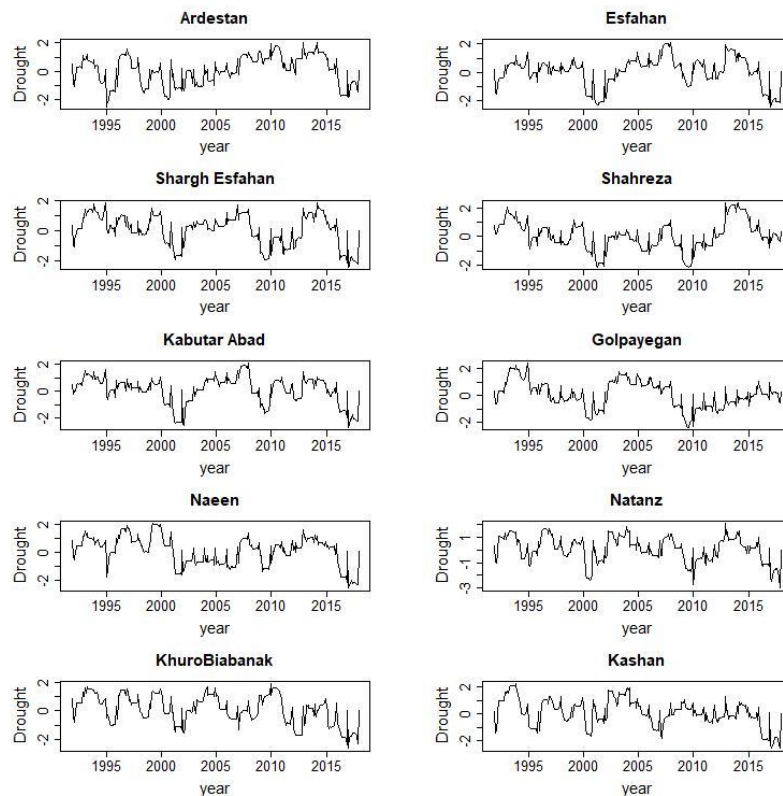
شکل ۸- سری های زمانی ( SPI_{24} ) کل ایستگاه های همیدی استان اصفهان.
