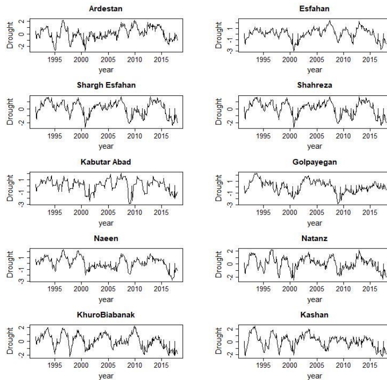
شکل ۷- سری های زمانی ( SPI_{18} ) کل ایستگاه های همیدی استان اصفهان.
