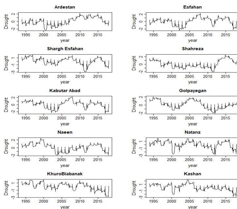
شکل ۹- سری‌های زمانی ( SPI_{(8)} ) کل ایستگاه‌های همدیدی استان اصفهان.
