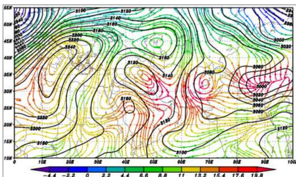
شکل ۲۲. نقشه ترکیبی ارتفاع ژئوتانسیل و وزش دمایی سطح ۷۰۰ هکتوپاسکال در موج ابر گرم
