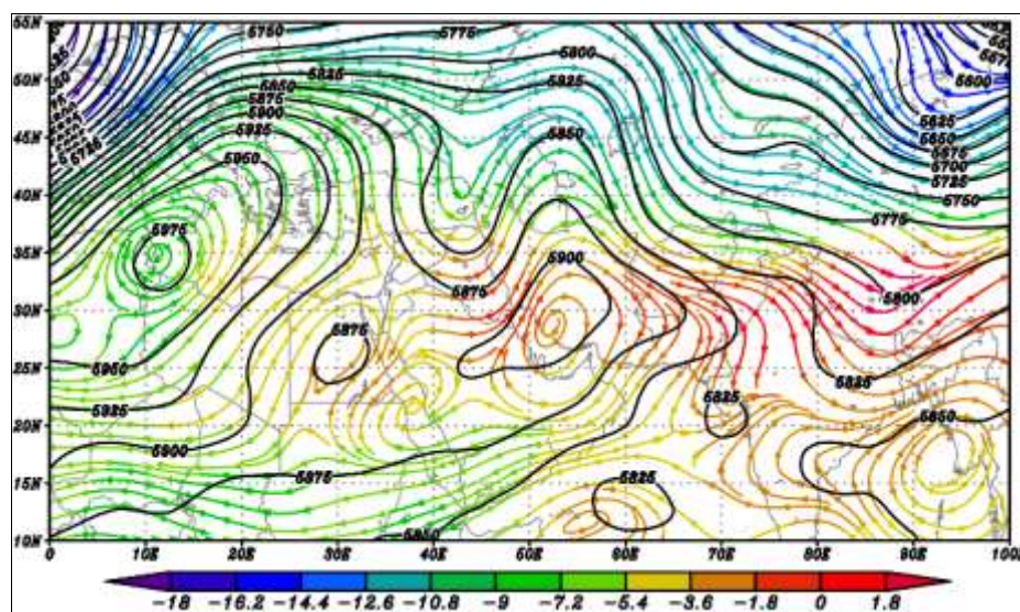
شکل ۲۱. نقشه ترکیبی ارتفاع ژئوتانسیل و وزش دمایی سطح ۵۰۰ هکتوپاسکال در موج ابر گرم
