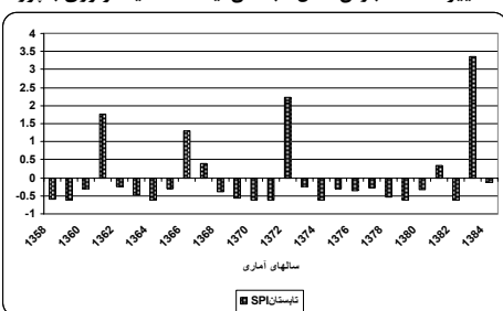
تغییرات SPI بارش فصل زمستان ایستگاه کیماتولوژی بمپور
