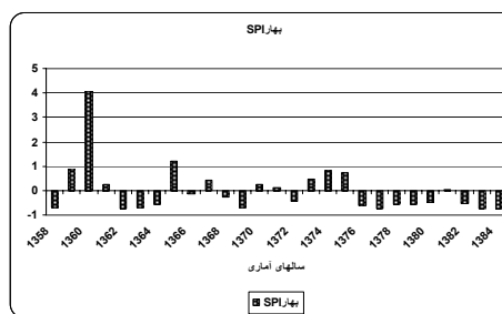
تغییرات SPI بارش فصل بهار ایستگاه سینوپتیک ایرانشهر
