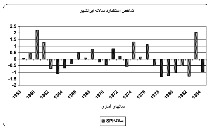
شکل شماره ۱: تغییرات SPI بارش سالانه ایستگاه سینوپتیک ابرانشهر
