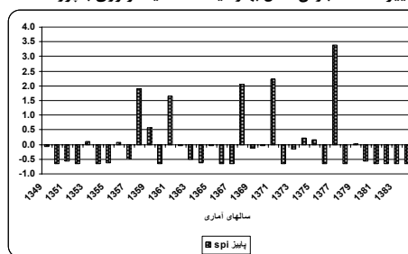
تغییرات SPI بارش فصل پاییز ایستگاه کیماتولوژی بمپور
