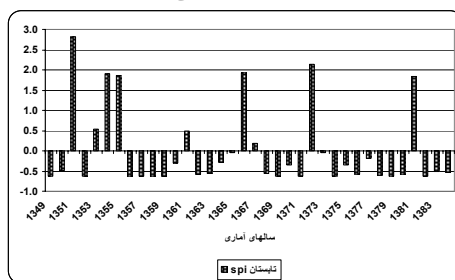
تغییرات SPI بارش فصل تابستان ایستگاه کیماتولوژی بمپور
