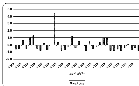
تغییرات SPI بارش فصل بهار ایستگاه کیماتولوژی بمپور
