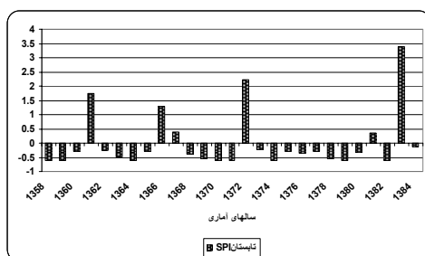
تغییرات SPI بارش فصل تابستان ایستگاه سینوپتیک ایرانشهر
