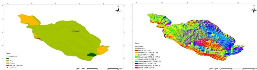
شکل (۴). جهت شیب حوضه آبخیز فیروزآباد شکل (۵). لیتولوژی حوضه آبخیز فیروزآباد
