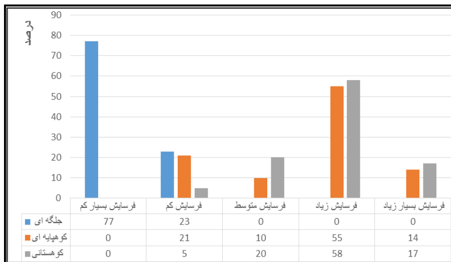
شکل (۵). سطوح فرسایشی به تفکیک لندفرمها در حوضه سفیدرود. مآخذ: یافته های محقق
