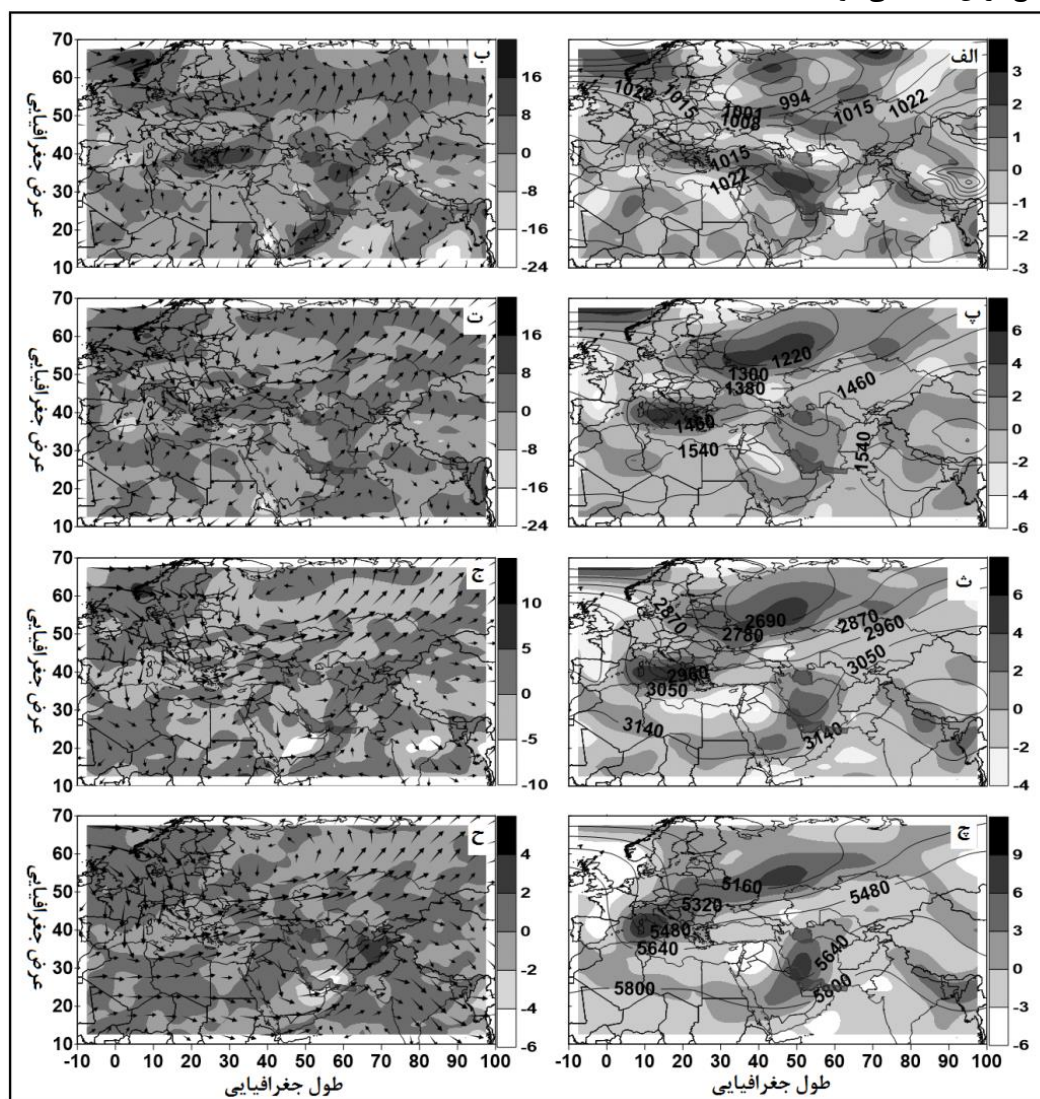
شکل (۵) نقشه (الف): فشار تراز ۱۰۰۰ هکتوپاسکال و تاوایی متر بر ثانیه ( 5 \times 10^{-5} s -1 ). نقشه (ب): همگرایی رطوبت تراز ۱۰۰۰ هکتوپاسکال بر حسب گرم بر کیلوگرم و جریان باد بر حسب متر بر ثانیه. نقشه (پ): ارتفاع تراز ۸۵۰ هکتوپاسکال بر حسب ژئوپتانسیل متر و تاوایی متر بر ثانیه ( 5 \times 10^{-5} s -1 ). نقشه (ت): همگرایی رطوبتی تراز ۸۵۰ هکتوپاسکال بر حسب گرم بر کیلوگرم و جریان باد بر حسب متر بر ثانیه. نقشه (ث): ارتفاع تراز ۷۰۰ هکتوپاسکال بر حسب ژئوپتانسیل متر و تاوایی متر بر ثانیه
