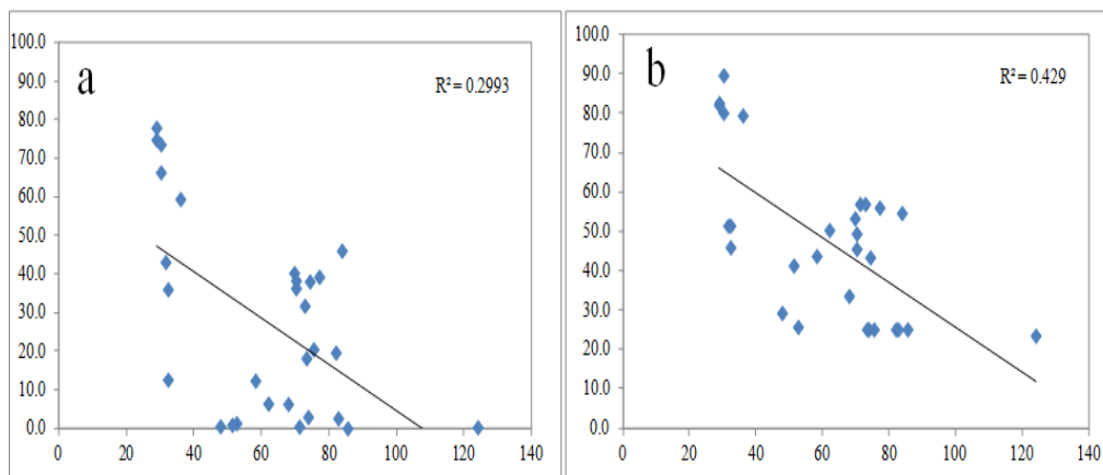
شکل (۱۰) همبستگی داده‌های پوشش برف و دی: (a) مادیس (b) MOD-AE
