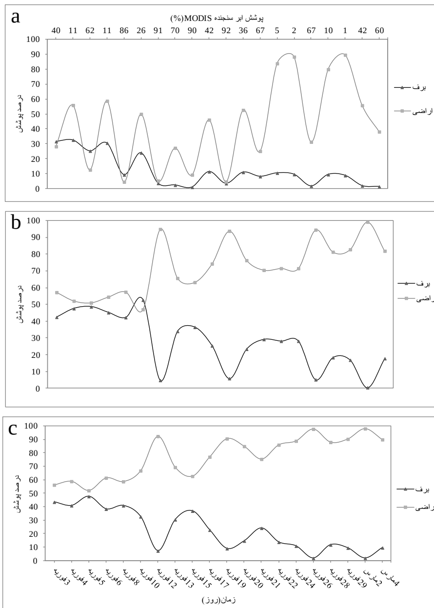
شکل (۶). درصد پوشش برف، اراضی و ابر، سال ۲۰۰۸: (a) MOD10A1، (b) AMSR-E و (c) MOD-AE
