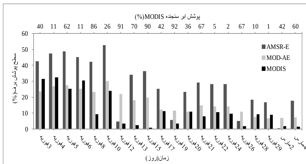
شکل (۸). تغییرات روزانه سطح پوشش برف پس از اعمال رابطه (۲)، سال ۲۰۰۸
