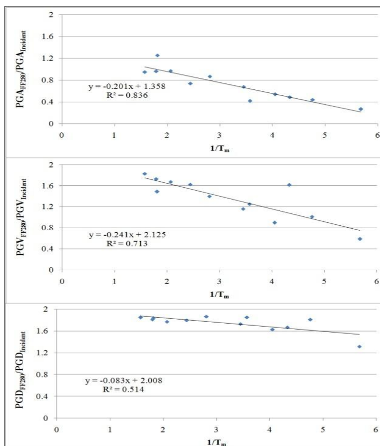
شکل ۷. نسبت بزرگ‌نمایی شتاب، سرعت و جابه‌جایی حاصل از تحلیل میدان آزاد برای ساخت‌گاهی با ارتفاع ۲۸۰ متر از سنگ بستر در مقابل معکوس پریود میانگین با نسبت میرایی ۵٪
