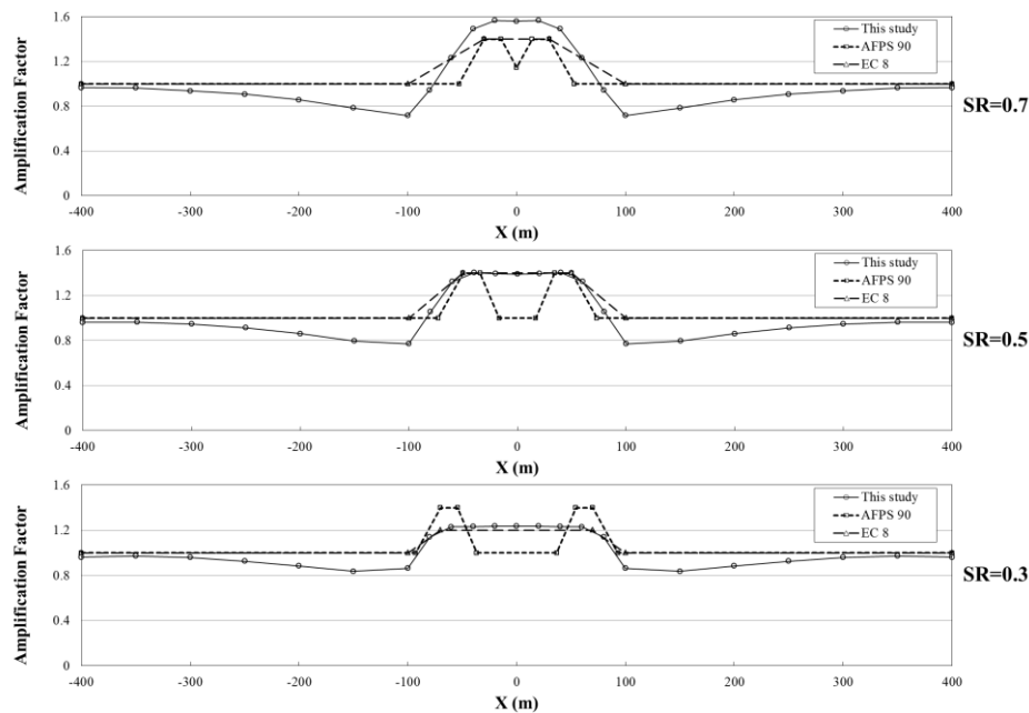
شکل ۱۳. مقایسه نتایج حاصل از تحلیل تپه دوزنقه‌ای شکل با نمودارهای حاصل از فرمول‌های تجربی AFPS ۹۰ و ضرایب پیشنهادی ارائه شده در EC ۸
