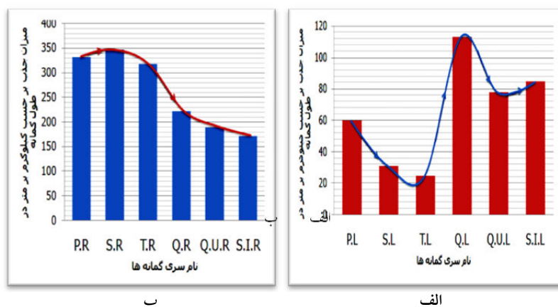
شکل ۴. الف) تغییرات جذب دوغاب در گمانه‌های سری اول تا ششم تکیه‌گاه راست سد البرز ب) تغییرات جذب دوغاب در گمانه‌های سری اول تا ششم تکیه‌گاه چپ سد البرز
