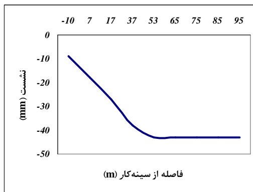
شکل ۷. جابه‌جایی در مقطع طولی تونل طولی تونل در مقطع بررسی شده
