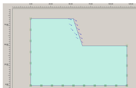
شکل ۳. نمایش تغییر شکل‌های کل برای تحلیل دوبعدی برای ترانشه به ارتفاع ۳۴ متر، شیب ۱ افقی: ۲ قائم و مصالح L1-1
