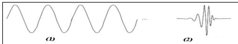
شکل ۱. مقایسه یک موج سینوسی (۱) با یک موجک (۲) ( 10\text{db} ).
