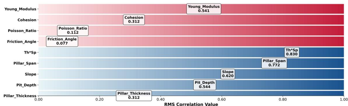
شکل ۴. میزان اثرگذاری پارامترهای ژئومکانیکی و هندسی لنگه تاج بر پارامترهای هدف بر اساس مجذور میانگین مربعات ضریب همبستگی Fig. 4. The influence of geomechanical and geometric parameters of the crown pillar on the target parameters based on the root mean square of the correlation value
