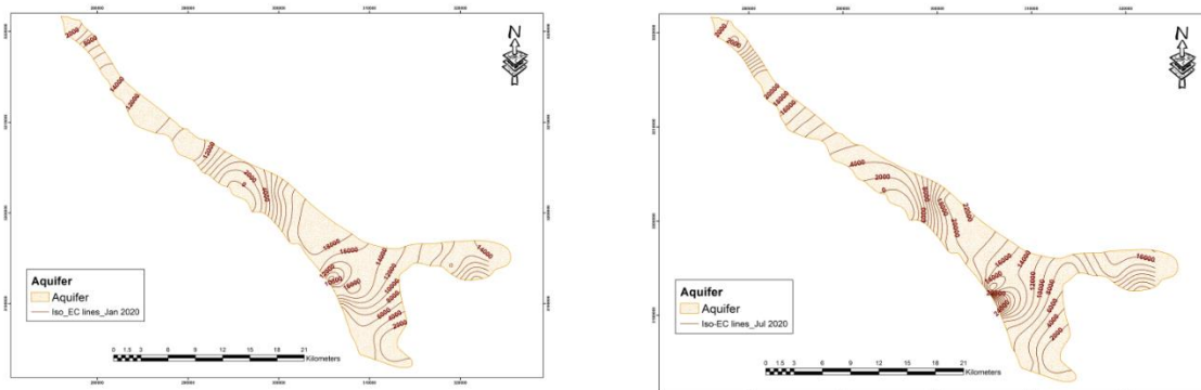
شکل ۸. خطوط هم هدایت الکتریکی آب زیرزمینی در زمستان ۱۳۹۸ (شکل سمت چپ) و تابستان ۱۳۹۹ (شکل سمت راست) بر حسب میکروموس بر سانتی‌متر در محدوده آبخوان
