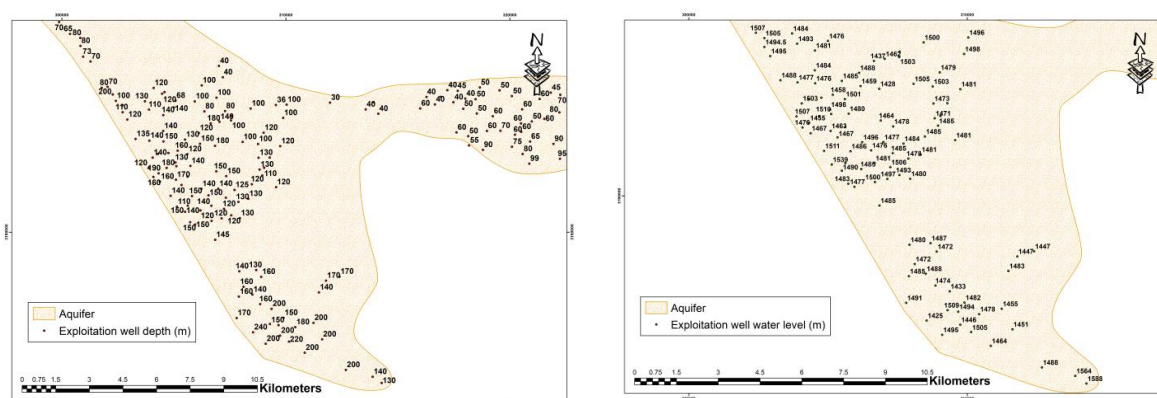
شکل ۱۲. موقعیت و عمق چاههای بهره‌برداری منطقه در بخش جنوب غربی آبخوان (شکل سمت چپ) و تراز سطح آب زیرزمینی چاههای بهره‌برداری با عمق بیش از ۹۰ متر در بخش جنوب غربی آبخوان (شکل سمت راست) بر اساس اطلاعات آخرین آماربرداری، اعداد بر حسب متر
