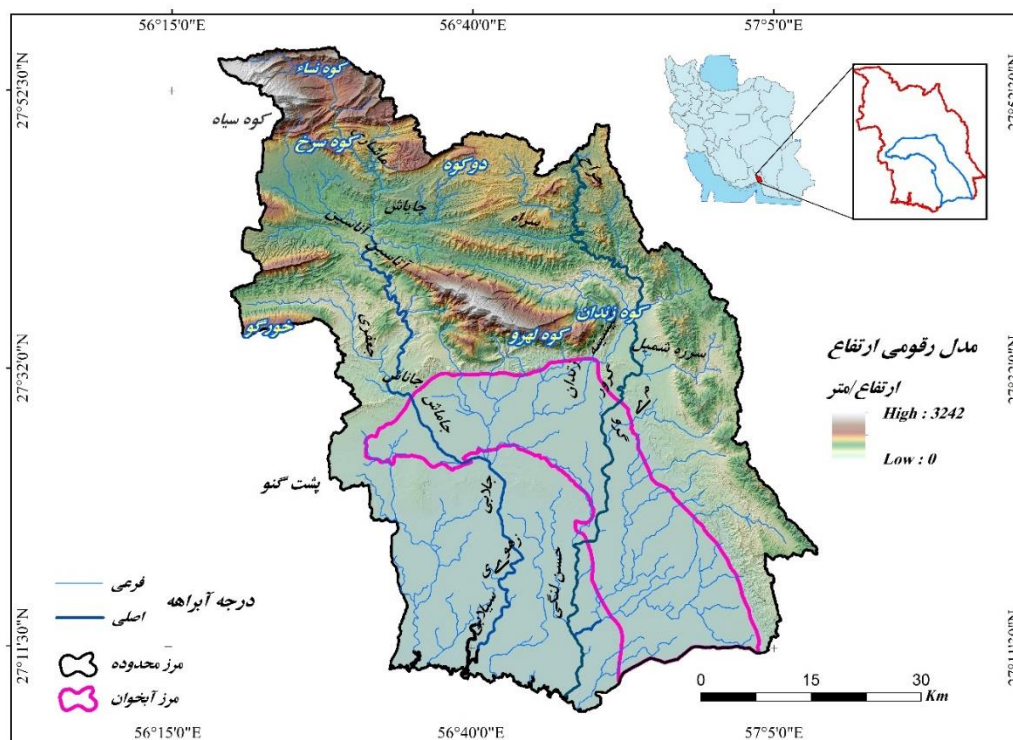
شکل ۱. موقعیت آبخوان شمل - تخت در محدوده مطالعاتی Fig. 1. Location of Shamil-Takht aquifer in the study area
