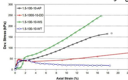
شکل ۶. نمودارهای تنش کرنش محوری ترکیبات ماسه و رس (1.5-100-10-WT;DD;WS;AP)
