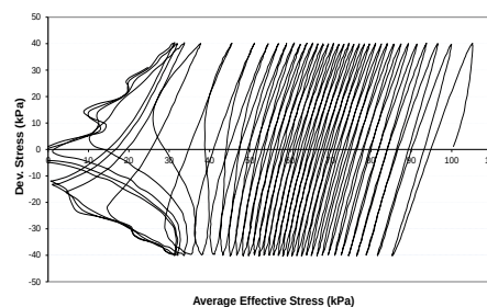
شکل ۱۸. مسیر تنش ترکیب 1.5-100-0-DD-0.2
