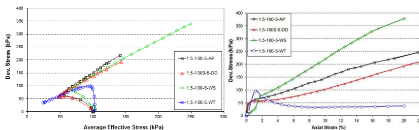
شکل ۴. نمودارهای تنش کرنش محوری ترکیبات ۵. نمودارهای مسیر تنش ترکیبات ماسه و رس (1.5-100-5-WT;DD;WS;AP) (1.5-100-5-WT;DD;WS;AP)
