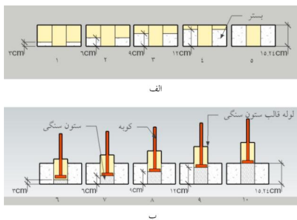
شکل ۸. شماتیک مراحل انجام آزمایش در دستگاه برش مستقیم الف) مراحل ساخت بستر، ب) مراحل ساخت ستون سنگی
