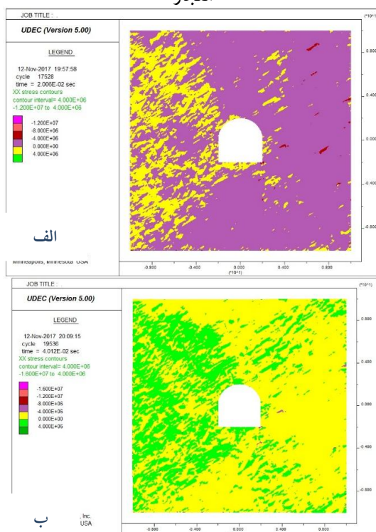
شکل ۱۳. کنتور تنش در راستای x ( S_{xx} ) در اطراف رمپ در مدت زمان الف) 20 میلی ثانیه، ب) 40 میلی ثانیه از اعمال بار دینامیکی انفجار
