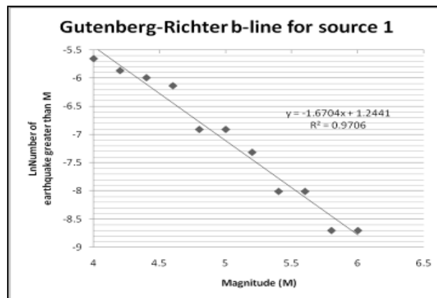
شکل ۷. نمودار گوتنبرگ - ریشتر، چشمه شماره یک
